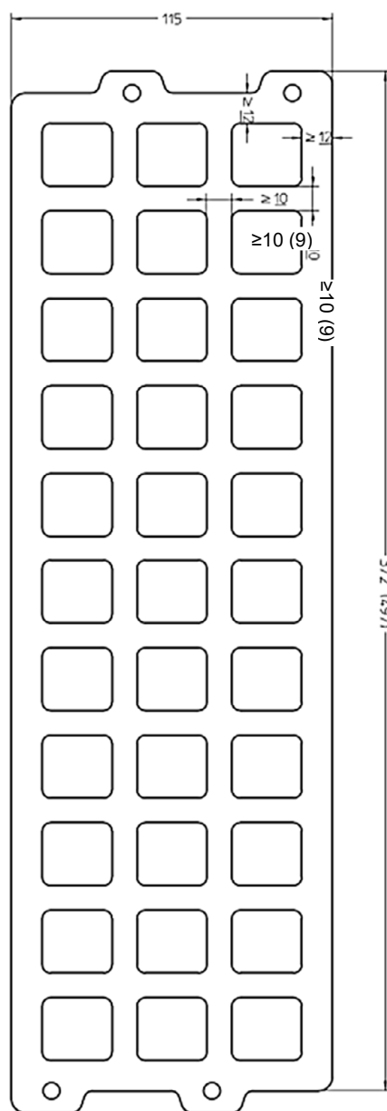
Maße und Stegdicken in mm
