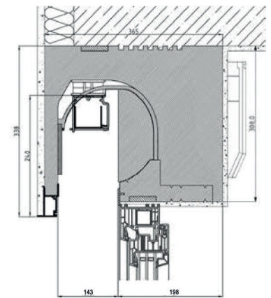
Revision Außen Jalousiekasten
