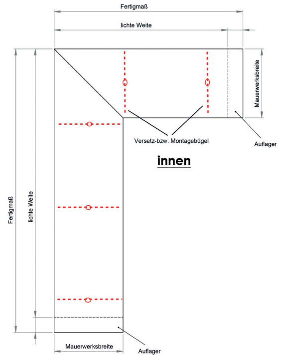
Gehrungsschnitt / Ecke (pro Schnitt)
