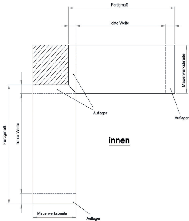
Eckschnitt (pro Schnitt)
