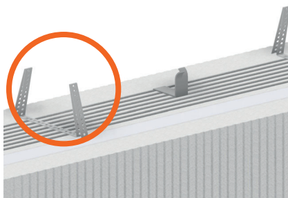
Lochband am Rollladenkasten vormontiert
