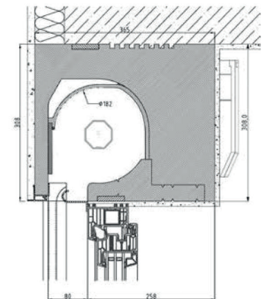
Revision Außen Rollladenkasten
