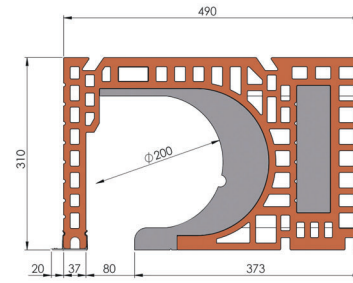
Klassik RG 49,0 Art.-Nr. 66 000 Gewicht 88 kg/m
