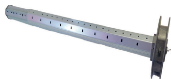
Teleskopwelle 60 mm Achteckwelle mit Walzenkappe, Teleskop und schiebbare Gurtscheibe Art.-Nr. 60 100
