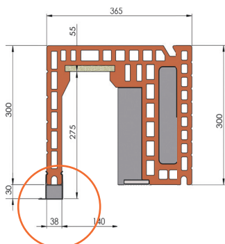
Jalousiekasten 36,5
