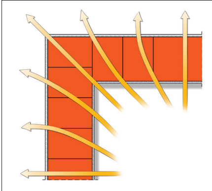
Bild 5.1: Wärmestromverlauf durch eine zwei-dimensionale, monolithische Außenwanddecke
